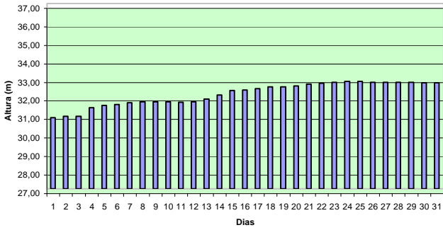
Dique Cruz del Eje - Mes: Marzo
