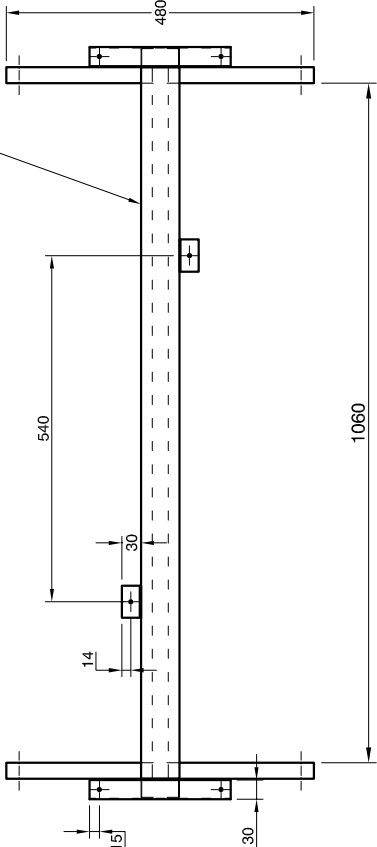
CAÑO ESTRUCTURAL 60x30x1.2mm
